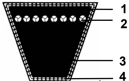
Узкоклиновой ремень
