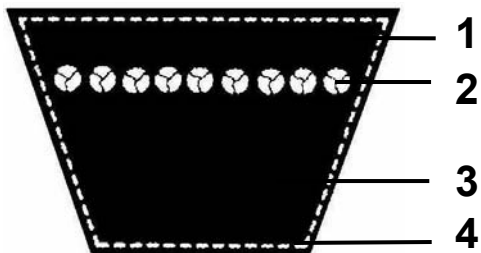
Классический клиновой ремень
